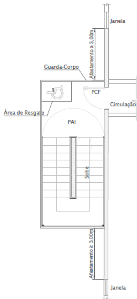
Figura 19 – Escada aberta externa.
