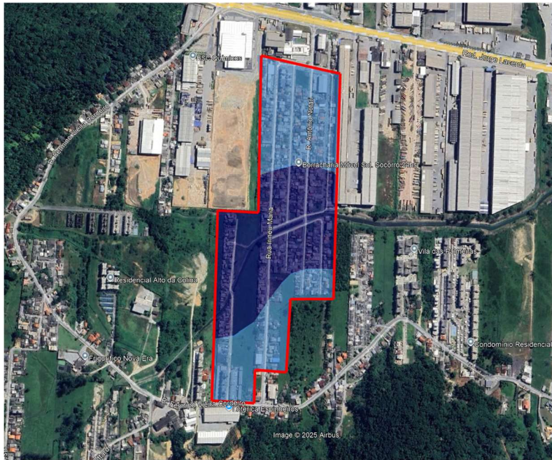
Figura 2. Áreas em azul escuro com nível de 1m de água (apenas embarcação), áreas em azul claro com 0,50m (permite acesso de veículos altos).
