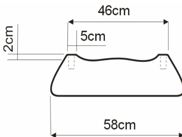
Corte A-A
